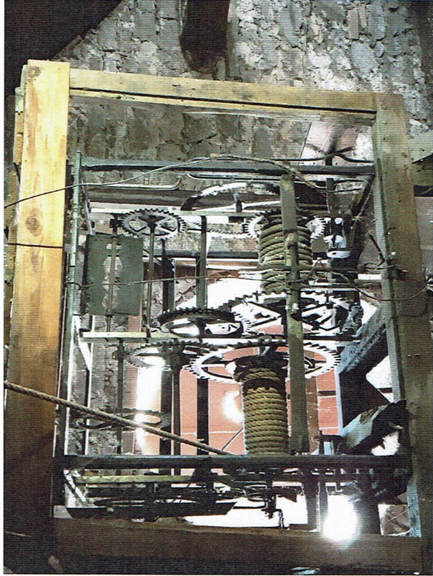
Vue générale de l'horloge du Château de Lassus
